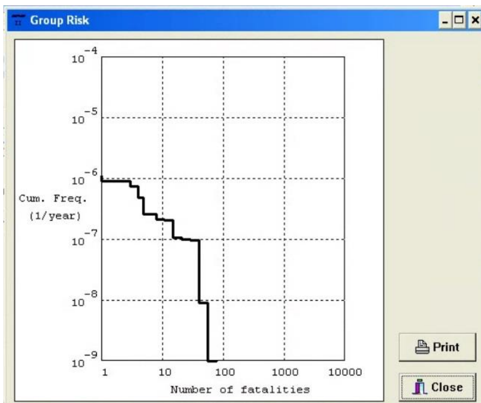
F-N görbe
