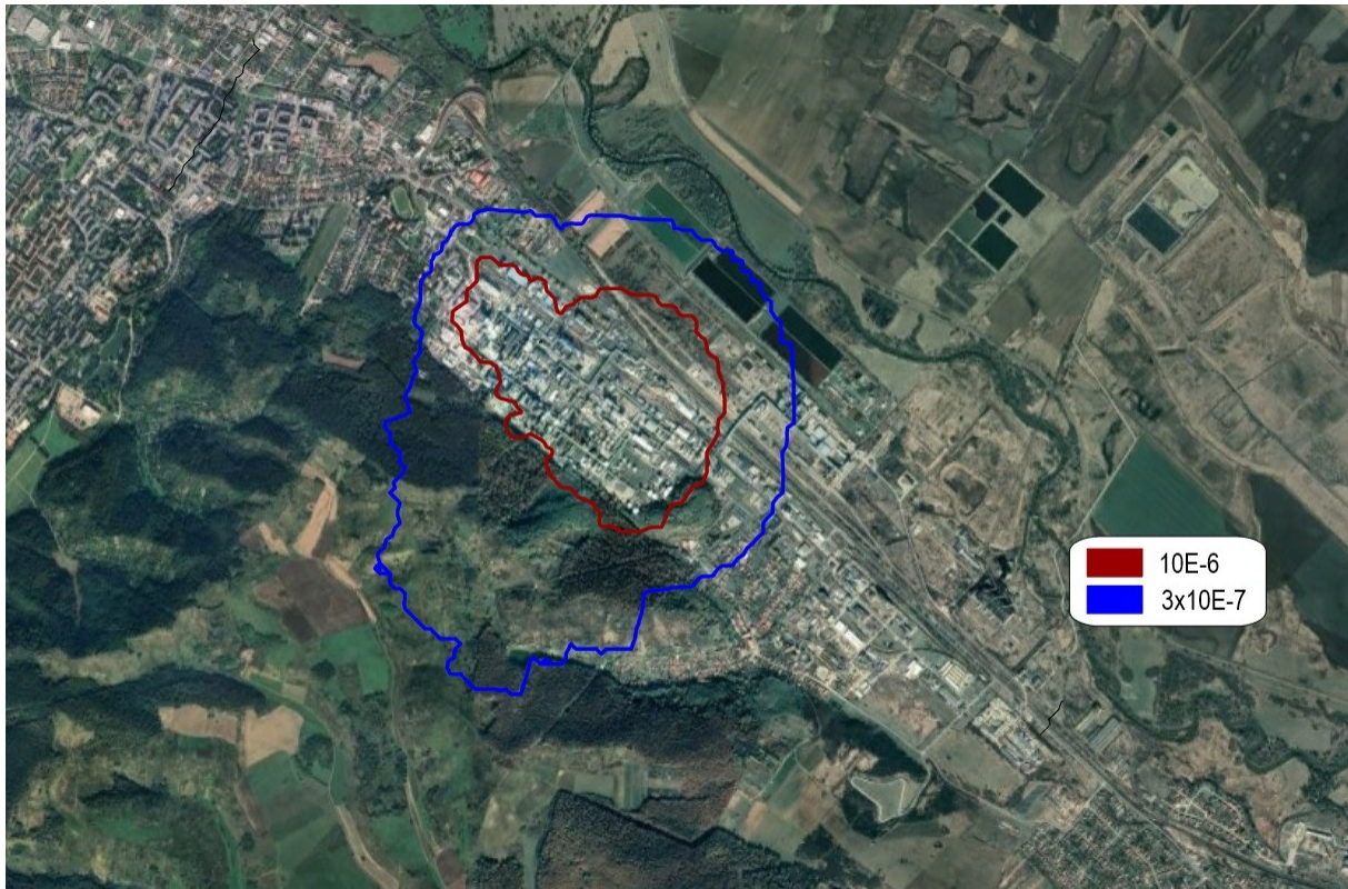
A BorsodChem Zrt. tevékenységéből származó aktualizált sérülés egyéni kockázati görbéi
