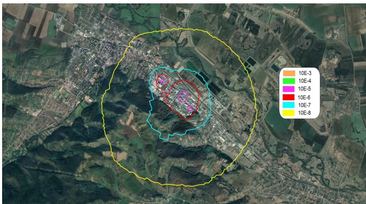
A BorsodChem Zrt. aktuális összesített egyéni halálózási kockázata
